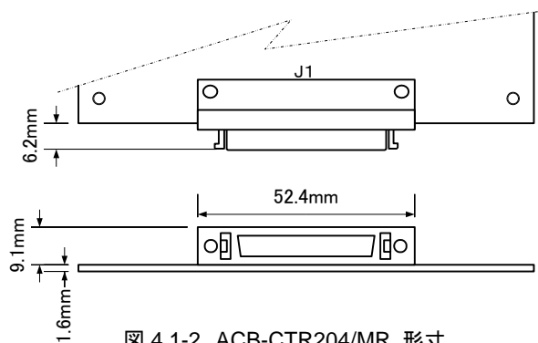
図 4.1-2 ACB-CTR204/MR 形寸
