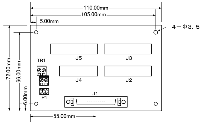
図 4.1-1 ACB-CTR204/MS 形寸
