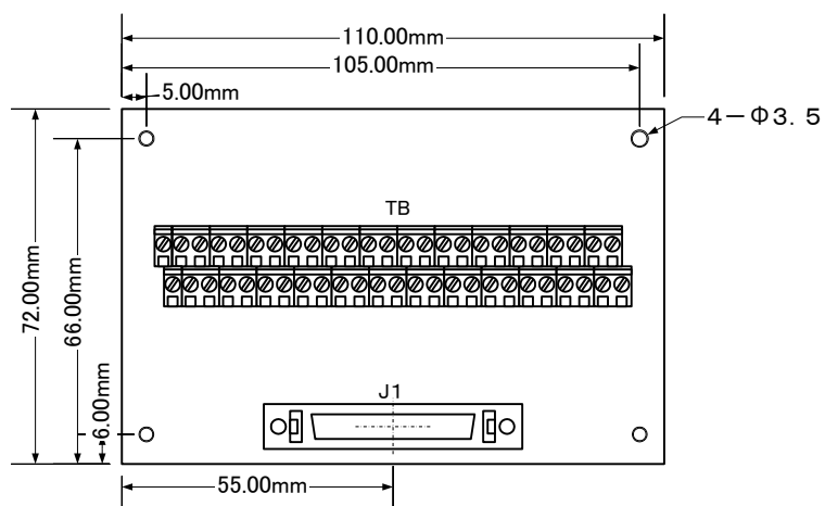
図 4.1-4 ACB-MDR50/MS 形寸
