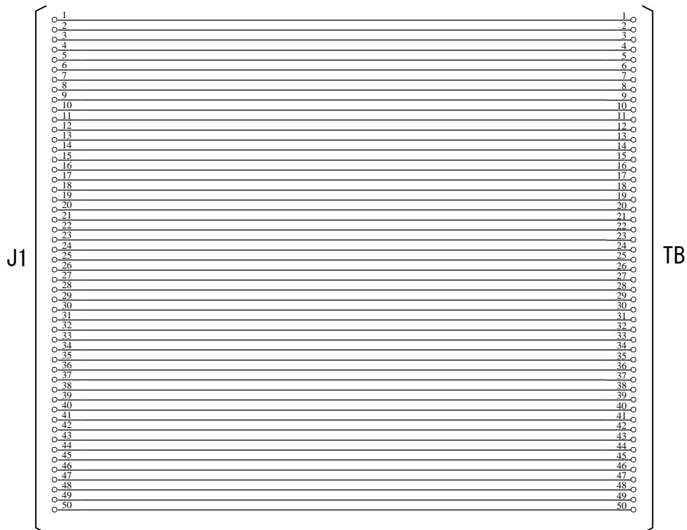
図 4.1-6 ACB-MDR50/ * 回路図
