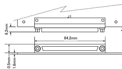
/DR 寸法図
