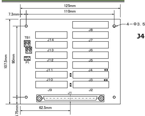
/DS,/DS(D)寸法図
