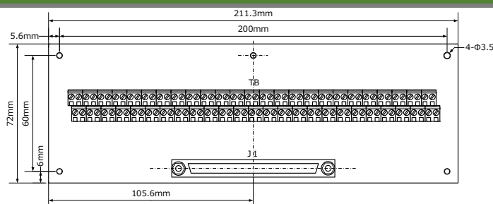
/DS,/DS(D)寸法図
