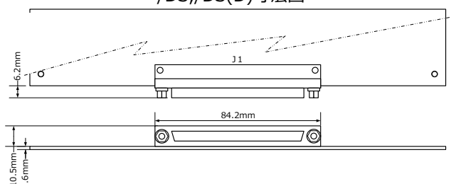
/DR 寸法図
