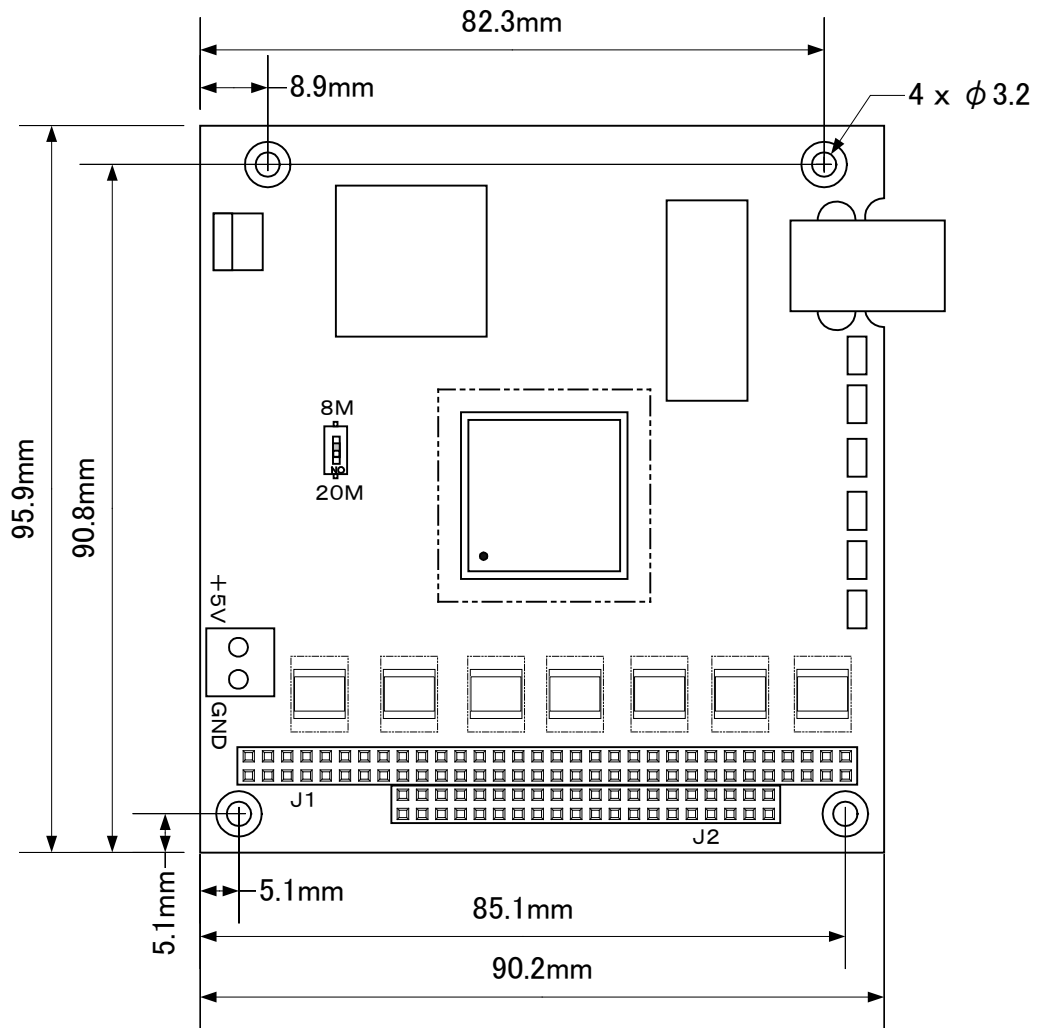
图 3.5-1 基板寸法图
