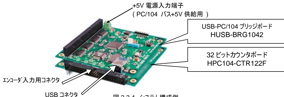
図 2.3-1 システム構成例
