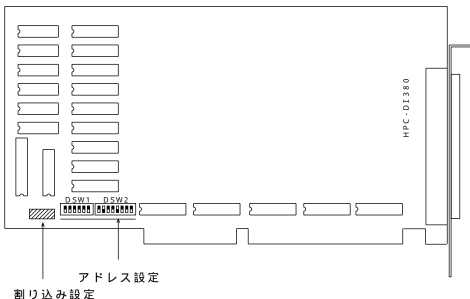
図3.1 ディップスイッチ及びジャンパの位置
