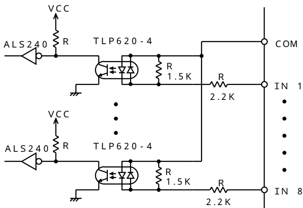
図 2.2 入力回路
