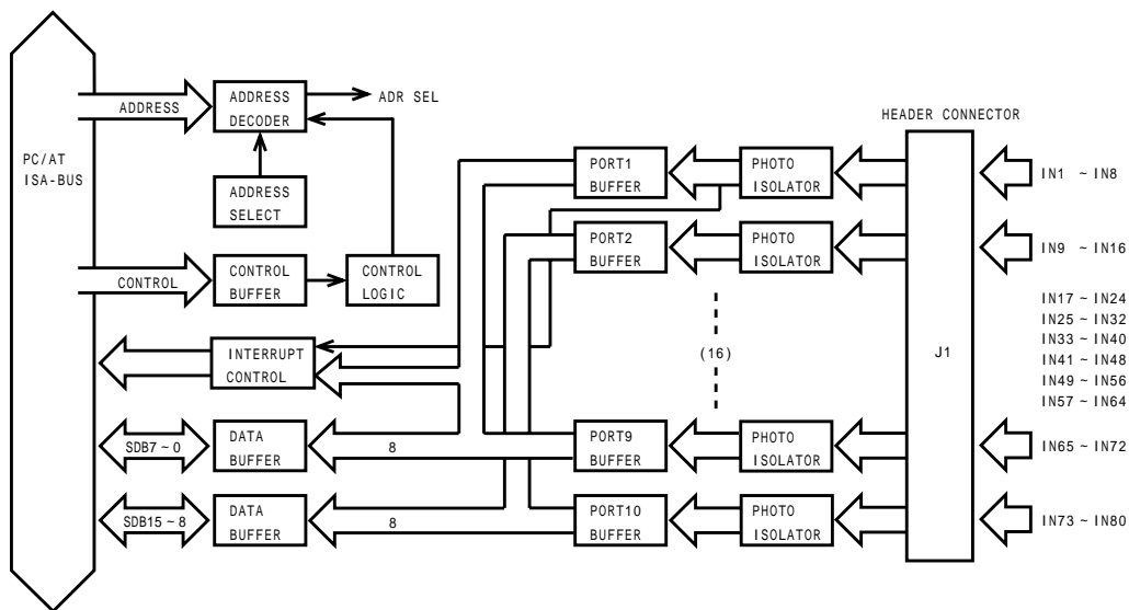
図 2.1 ブロックダイヤグラム
