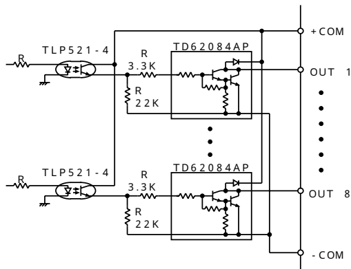
図 2.3 出力回路
