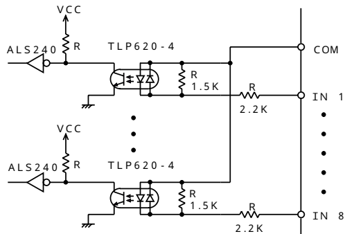
図 2.2 入力回路
