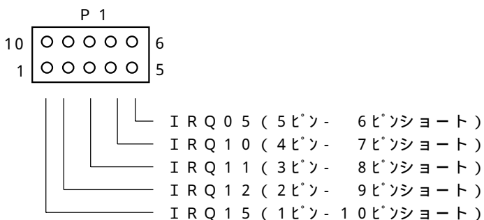
図 3.5 ジャンパ端子接続位置
